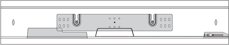
gabarit d'installation pour montage au mur
